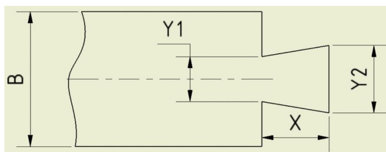
Schwalbenschwanzgeometrie
