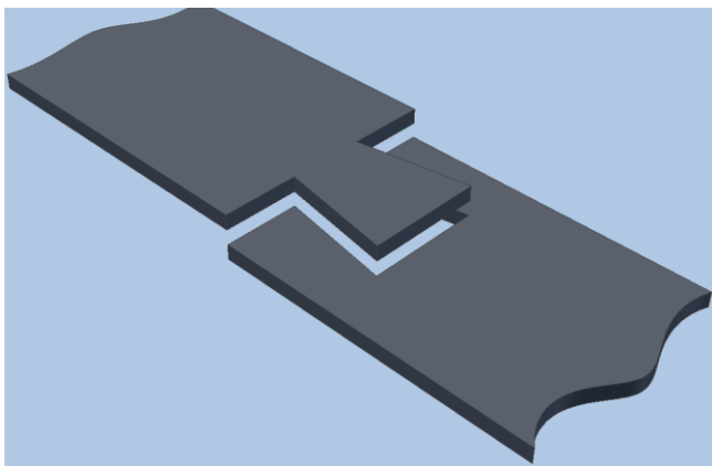
Schwalbenschwanz
