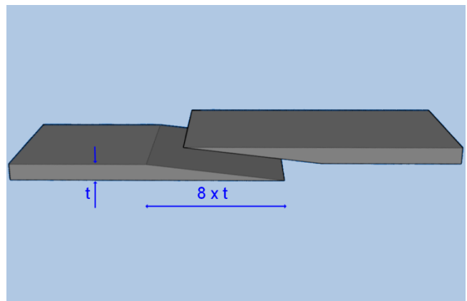
Schäften
